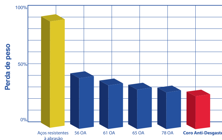
Teste de desgaste abrasivo ASTM G65
